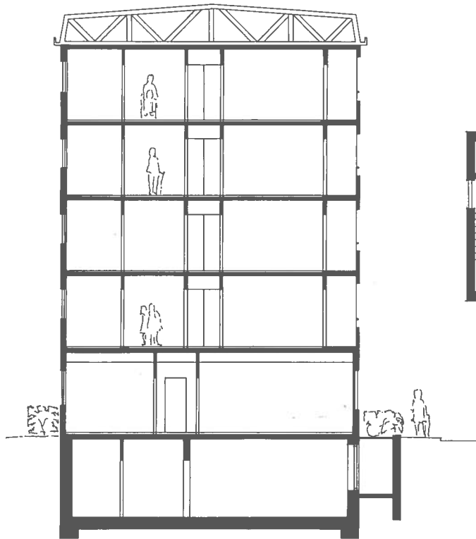
Snit 1:200
