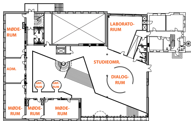
STUEPLAN
