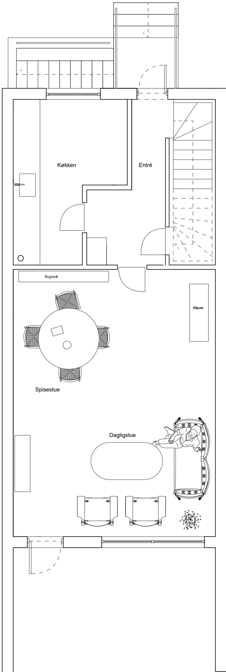
Eksisterende plantegning
