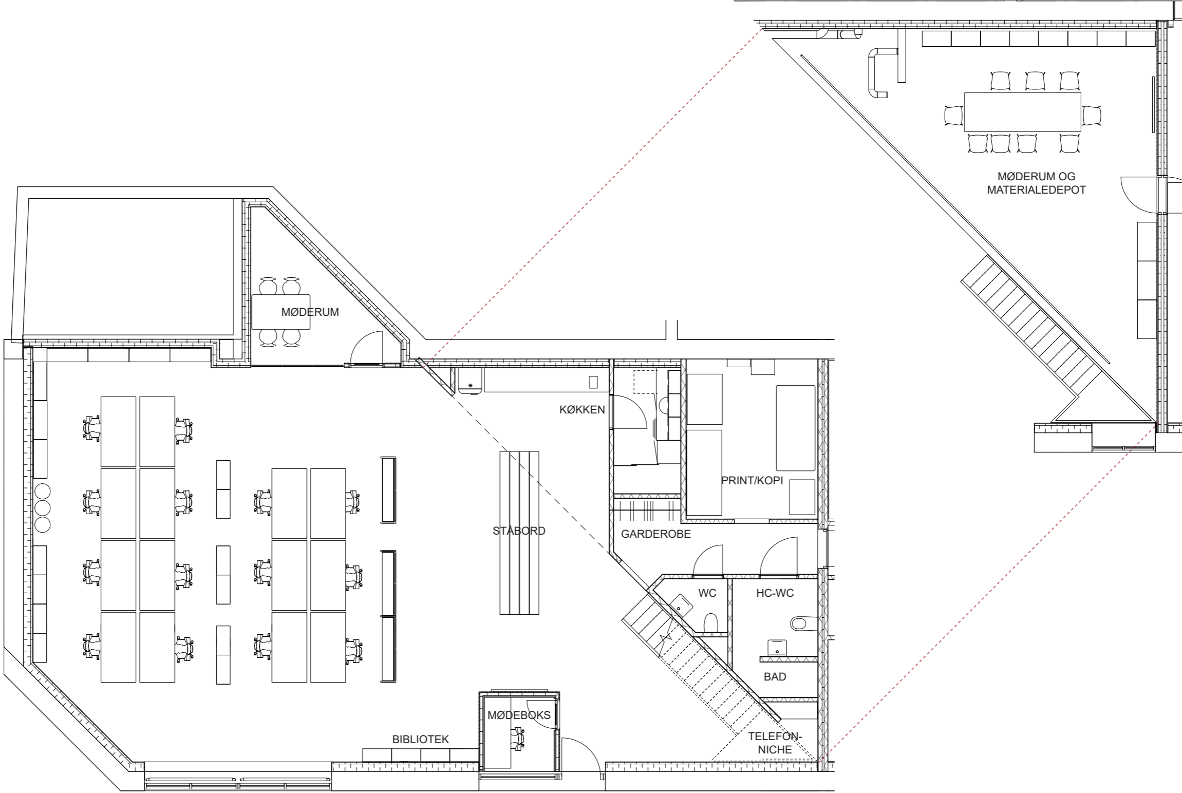
STUEPLAN
