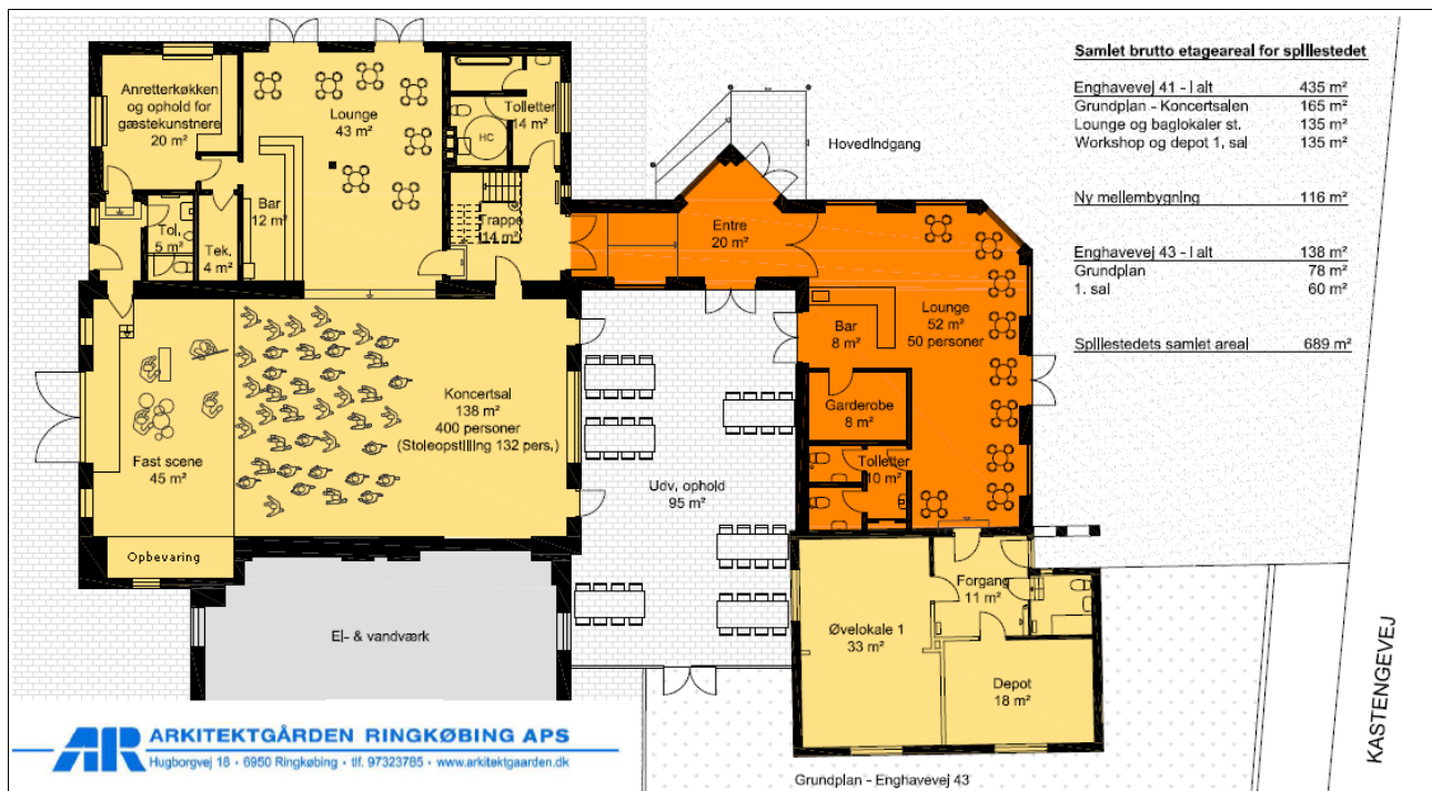
Fig. 1: Grundplan. Gule arealer er eksisterende forhold, som renoveres og ombygges. Orange område er nybygning som forbinder de eksisterende bygninger
