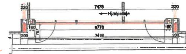
Delplan af stålkonstruktion 1 : 75
