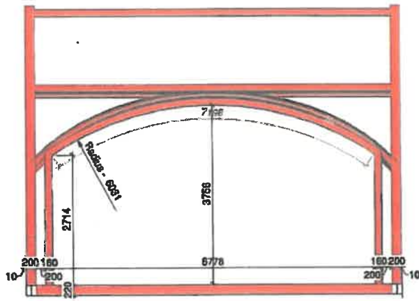
Front af stålkonstruktion
