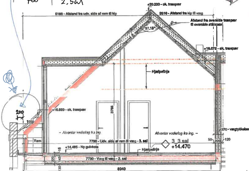
Snit i bue 1 : 50
